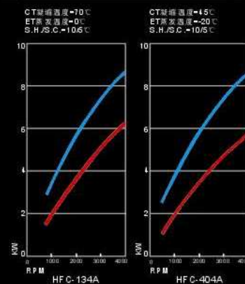
HCP-19 Performance Curve 性能曲线
