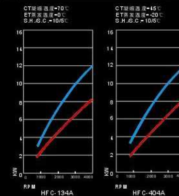
HCP-23 Performance Curve 性能曲线
